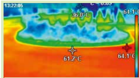
A hőkamerás felvételen jól kivehető az aszfaltozott és a zöldterület közötti hőmérsékletkülönbség
